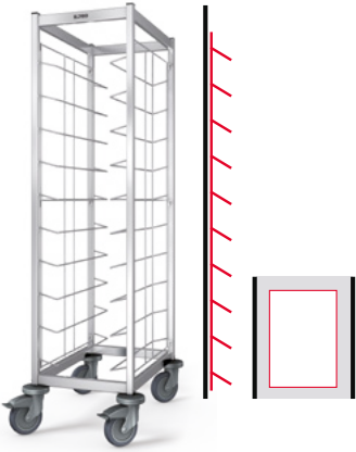
10 Auflagen mit je 125 mm Abstand, Tabletteinschub längs
